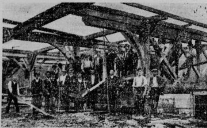
Postavljanje poda ali kozoleca je po naših vaseh vedno vesel dogodek. Ker je posebniku Pevcaču na Jagnjenici strela uničila skedenj, mu je mojster Blaj iz Radeč napravil novega, katerega so številni sosede pomagali postaviti
