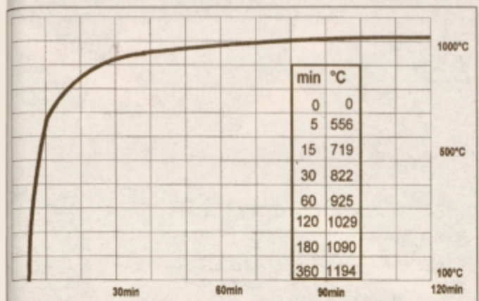
Slika 2 Naraščanje temperature okolice v primeru požara
