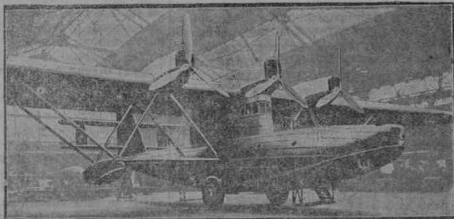
Novi noriška motorna ladja za prevažanje petroleja. Ladja ima 18.000 ton, dolga je 165 m, gre 9 m lahko globoko in sprejme 22.730 kubičnih m petroleja. — Desno: Novo prekoceansko letalo bo obratovalo na progi Paris-Njujork.
