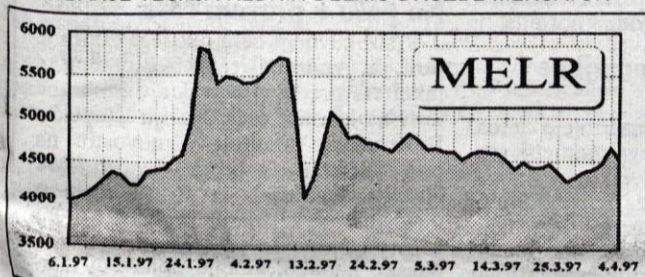
GIBANJE TEČAJA REDNIH DELNIC DRUŽBE MERCATOR
