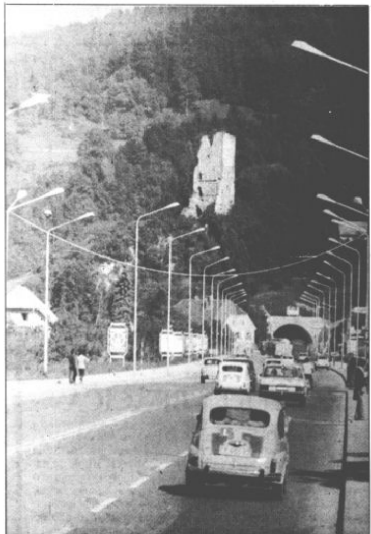
V sredo smo v Velenju izročili namenu še eno pomembno pridobitev: nov cestni predor pod razvalino Šaleškega gradu in odsek asfaltirane ceste do Sela. Predor, ki so ga gradili delavci REK Zasavje, tozdr rudarska gradbena dejavnost, je dolg skupaj z izvirno cevjo 93,4 metra, širok pa 9,6 metrov. Njegov investitor je bila samoupravna komunalna skupnost občine Velenje. Novi predor je izredno pomembna pridobitev, saj bo s prestavitvijo ceste odpravljeno ozko grlo skozi vas Salek, pridobili pa smo tudi nove preprote površine za stanovanjsko in drugo gradnjo. V primeru potrebe pa bo lahko služil tudi kot zaklon za tamkajšnje prebivalce.
