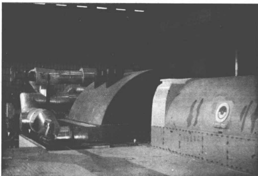
Novi turboagregat TEŠ IV: levo turbina, desno generator
