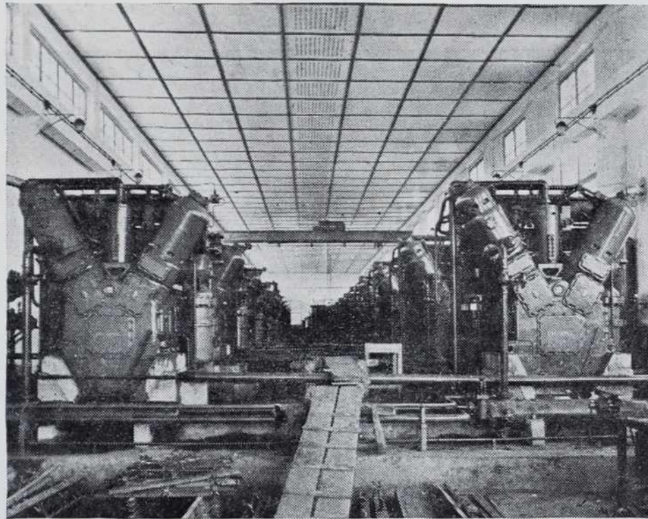
Pogled v veliko kompresorsko dvorano podjetja Nafta v Lendavi.
