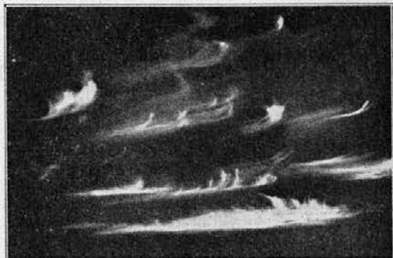
Cirus, oznanjevalec slabega vremena
