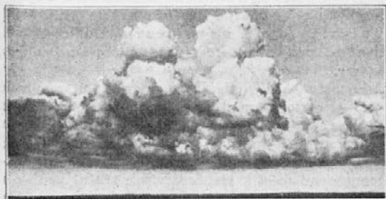
Kumulo - nimbus, oblak poletnih neviht
