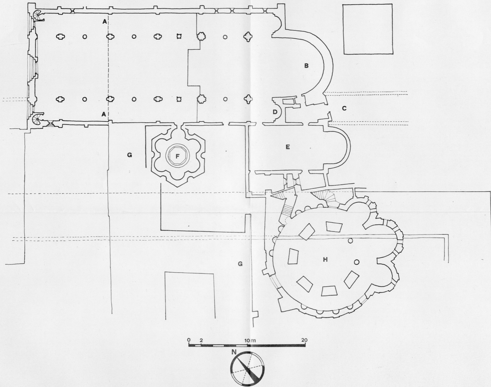
Fig. 1. Zadar (Zara). Complesso architettonico della Cattedrale: A. Facciata (primitiva della Cattedrale), B. Abside, C. Via romana, D. Abside meridionale con i resti del pavimento musivo primitivo, E. Sacrestia, F. Battistero, G. Episcopio, H. Chiesa di S n Donato
