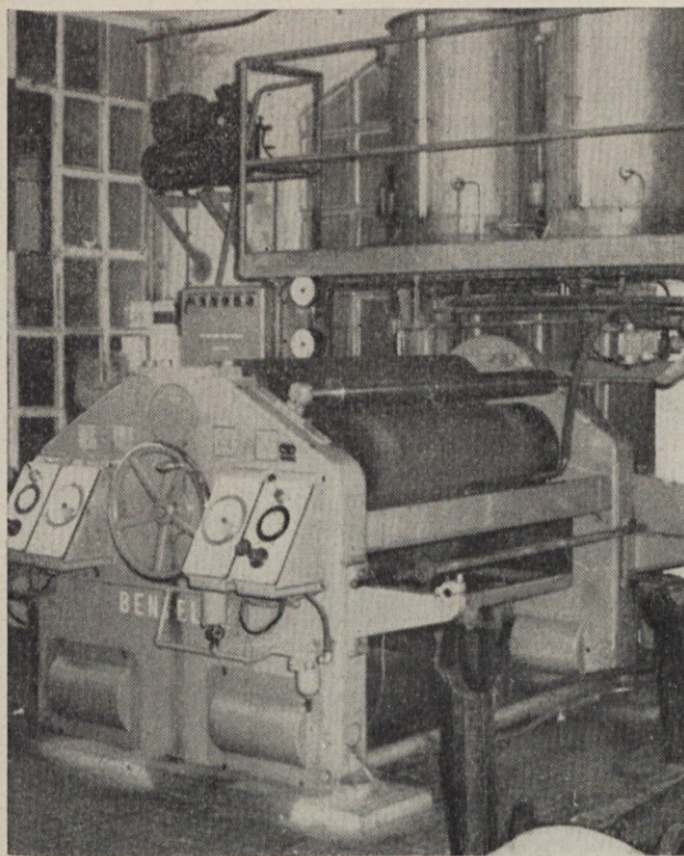
Foulard, s katerim smo izboljšali barvanje naših tkanin
