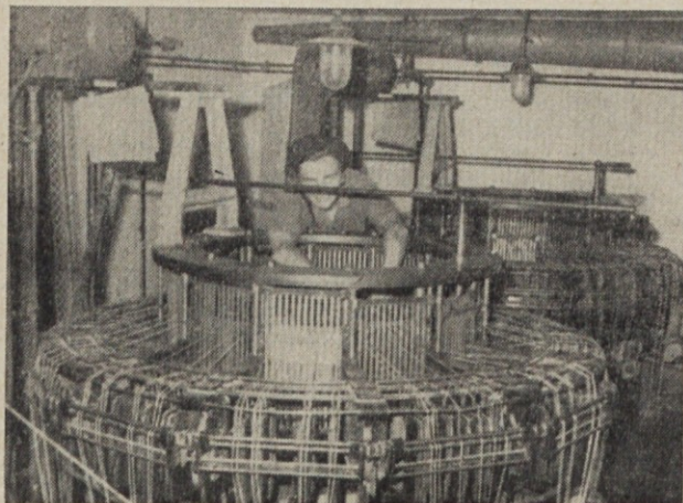
Stroji za okroglo tkanje gasilskih cevi
