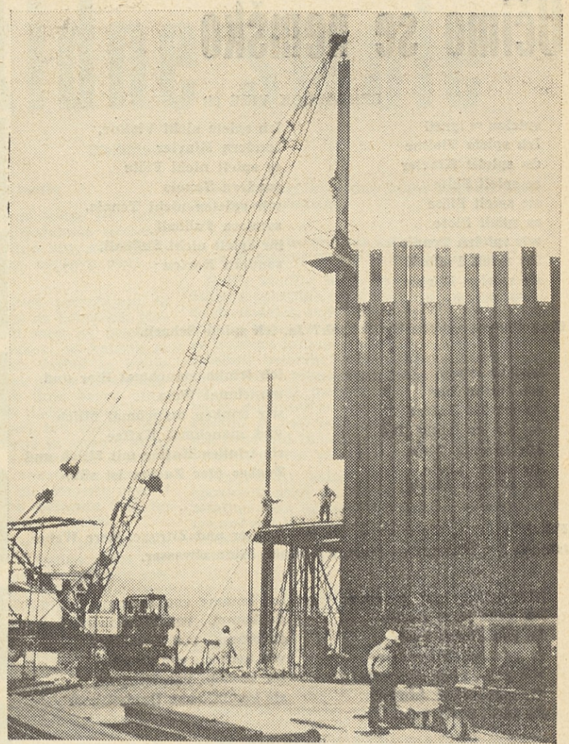
Pri gradnji petega naveza v Luki Koper je potrebno v osmih celicah zabiti 32.764 m Beval PBP zagatnic, tipa 9,5 in 853 metrov zagatnic tipa PBT, 915. Na sliki ob začetku del — zabijalo stoji pod pravkar dvignjeno zagatnico
