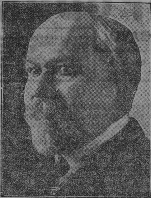
Poincare.
