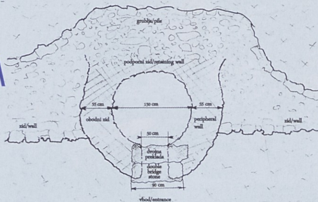
Tloris/ground plan: Hiška Ivanjki grad - Kras 07. 2013
