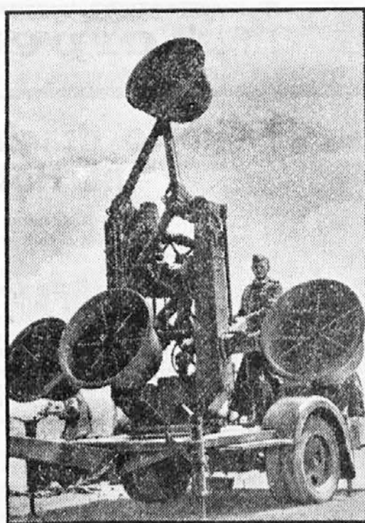
Priprava, ki naznanja Nemcem ob belgijski obali, da se bližajo angleška letala.
