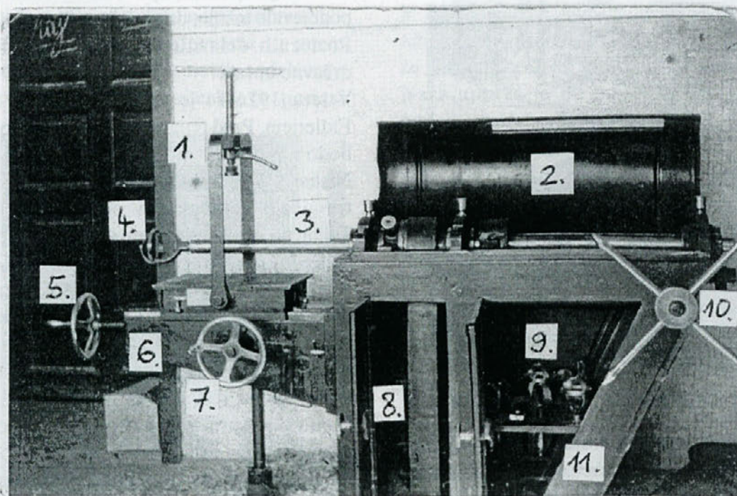
Vrtni stroj za izdelavo protez. Konstruiral Anton Jež 1926
