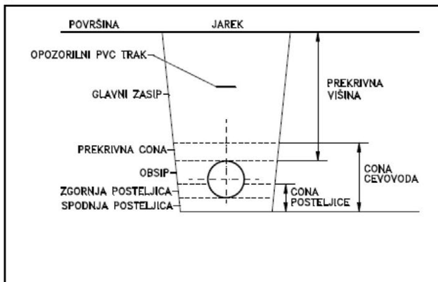
Slika 1: Prerez jarka
