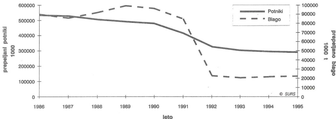
Slika 8: Potniški in blagovni promet, Slovenija, 1986-1995
