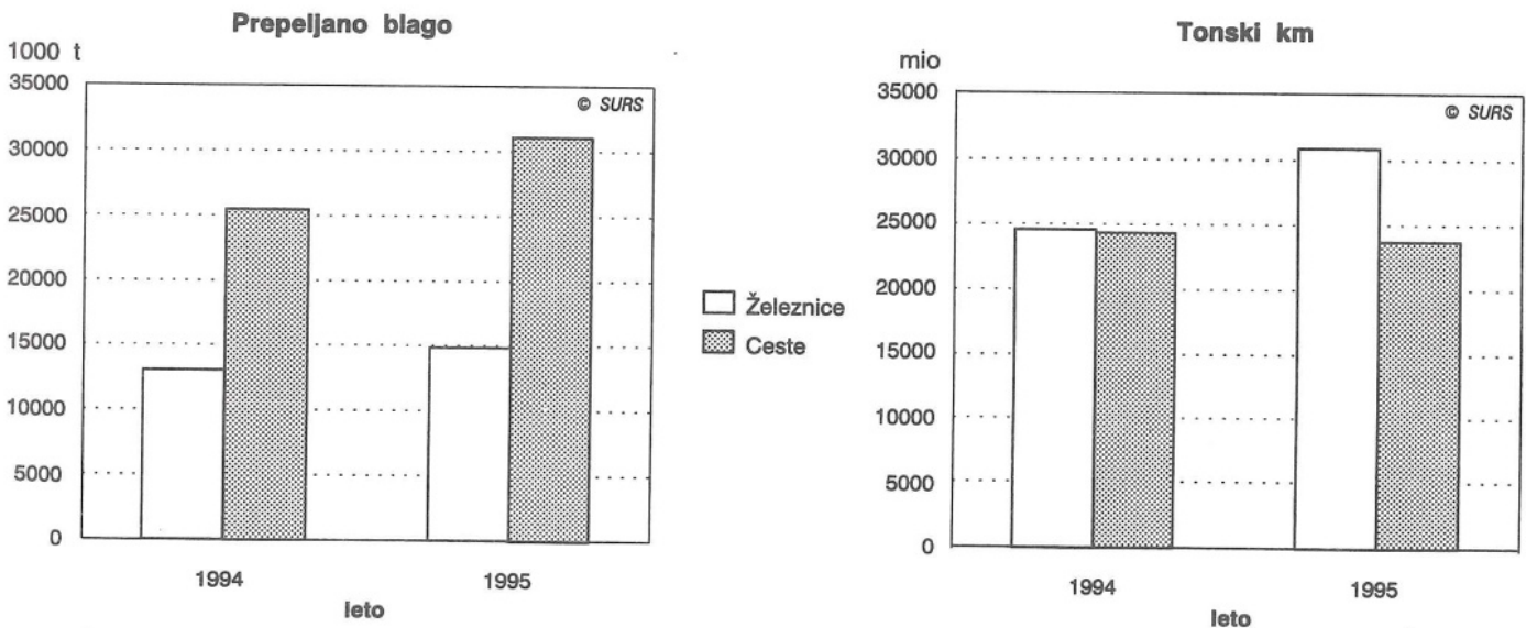
Slika 17: Železniški in cestni blagovni promet, Slovenija, 1994-1995
