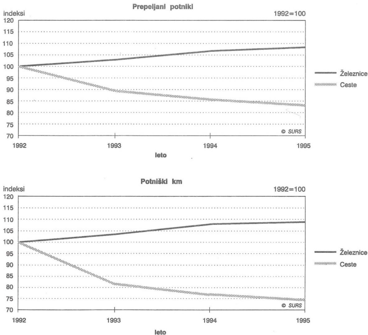
Slika 14: Kopenski potniški promet, Slovenija, 1992-1995
