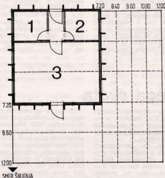
1. Pisarna 2. Sanitarni blok 3. Proizvodni prostor
