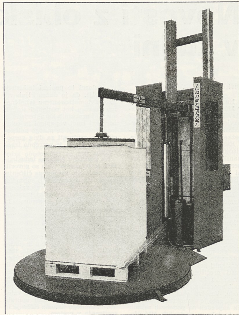
Stroj za avtomatsko zavijanje palete papirja v folijo
