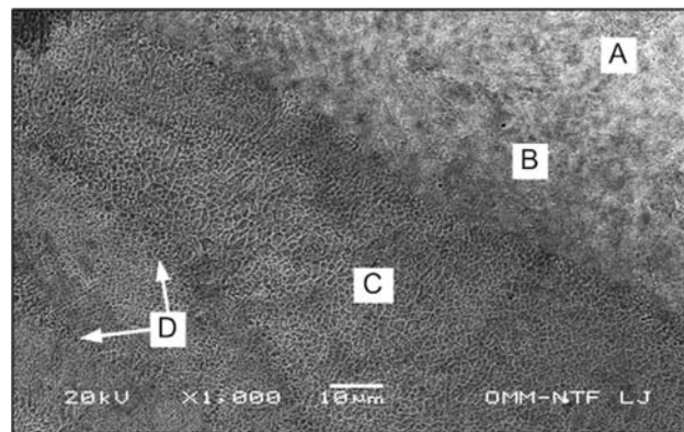
Slika 10: Mikrostruktura jekla na robu zvara: A-osnovni material; B-TVP; C-območje celično-dendritne mikrostrukture; D-pasovi toplotnega vpliva zaradi večvarkovnega polnjenja žleba; SEM (SEI)
