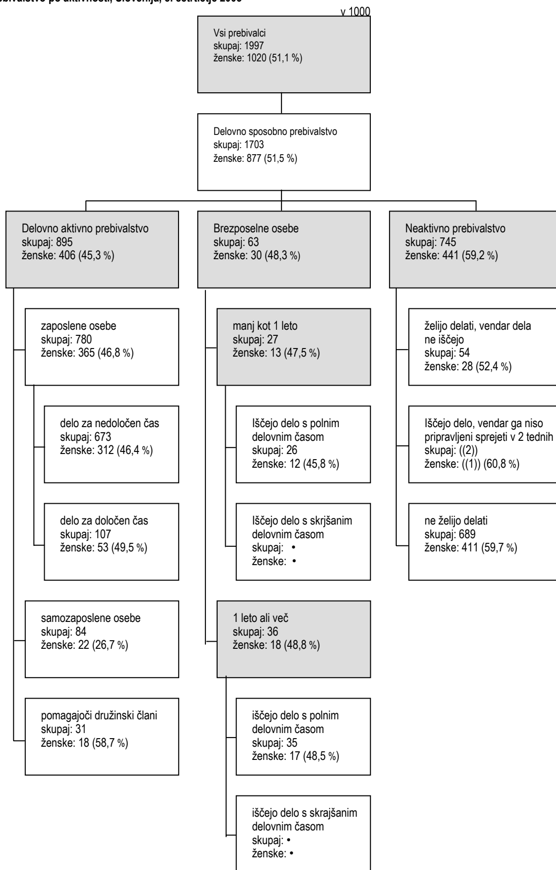
Slika 9: Prebivalstvo po aktivnosti, Slovenija, 3. četrletje 2003
