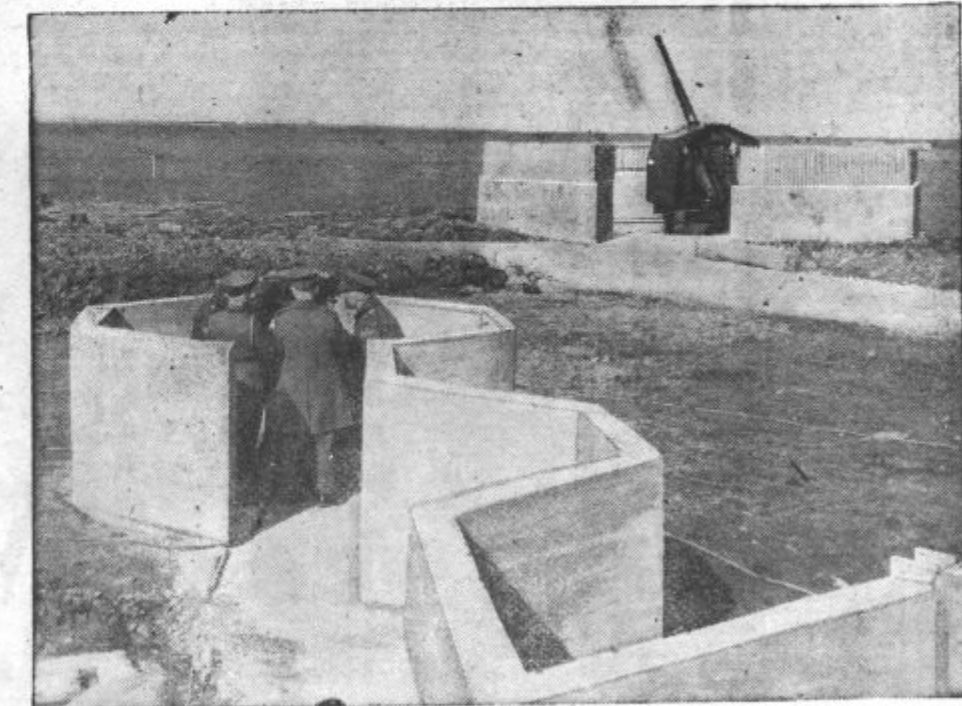
PROTILETALSKI TOPOVI V ANGLIJI. Angleške protiletalske straže imajo službo na posebnih postojankah iz železobetona
