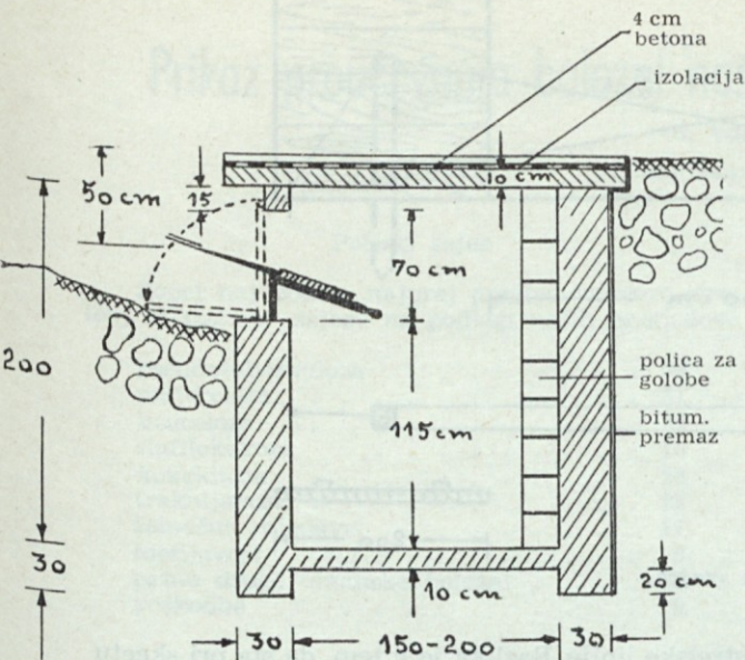
Rov za namestitev ročnih strojev za metanje glinastih golobov
