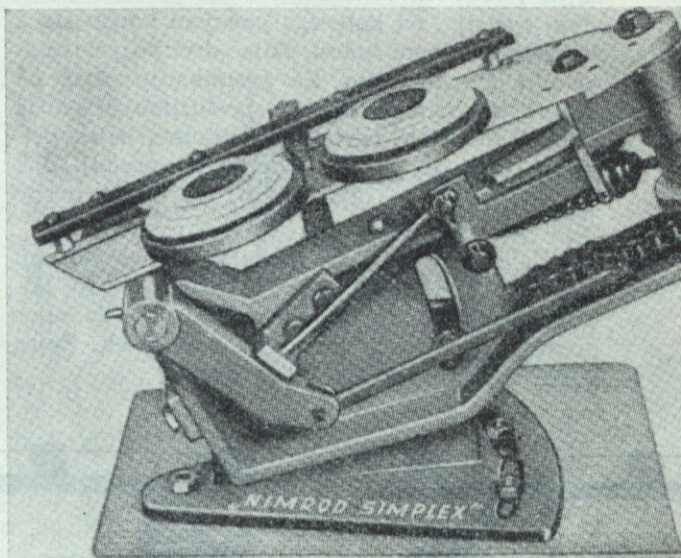
Sodoben stabilni stroj za metanje glinastih golobov z električnim proženjem, firme Nimrorodwerke
