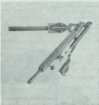
Ročni stroj za metanje glinastih golobov
