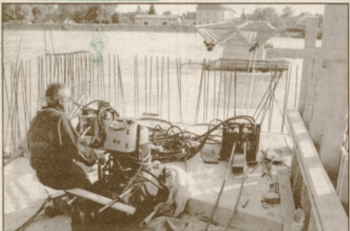
Več kot 120 ton težko jekleno konstrukcijo so na levi breg povlekli s pomočjo dveh hidravličnih naprav. Foto: M. Ozmeč
