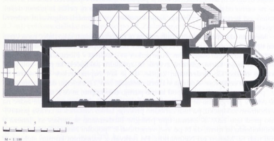
Slika 12: Ormož, župnijska cerkev sv. Jakoba st., poskus rekonstrukcije stanja v 13. stoletju. Risal: B. Vnuk, september 2004
