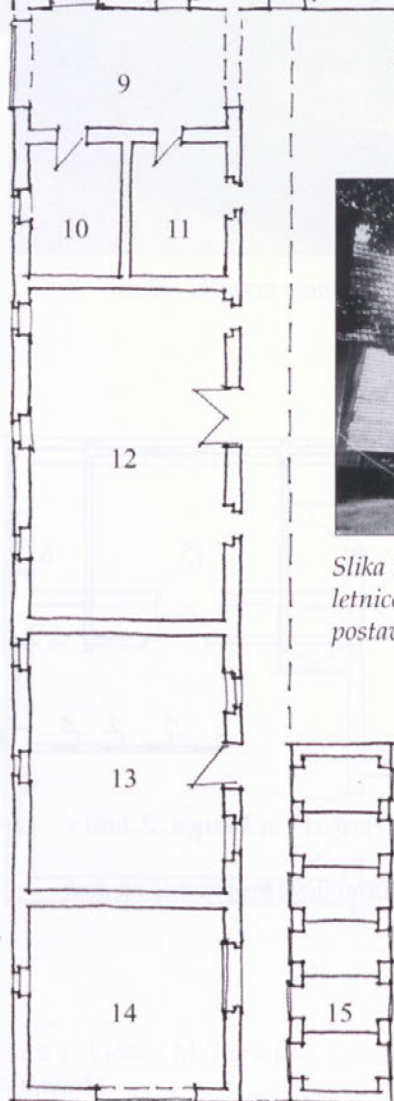
Skica 3: Rucmanci 57: Tloris hiše s pravokotno nanjo postavljenim gospodarskim poslopjem: 1. veža »priklet«, 2. kuhinja, 3. hiša s krušnico pečjo, 4. štiblc z ozkim delom krušne peči, 5. zadnja hiša s krušno pečjo (pred leti porušena), shramba, 7. shramba, 9. pokrit hodnik, 8. 10. 11. kleti, 12. hlev, 13. hlev, 14. gumno, 15. svinjak.
