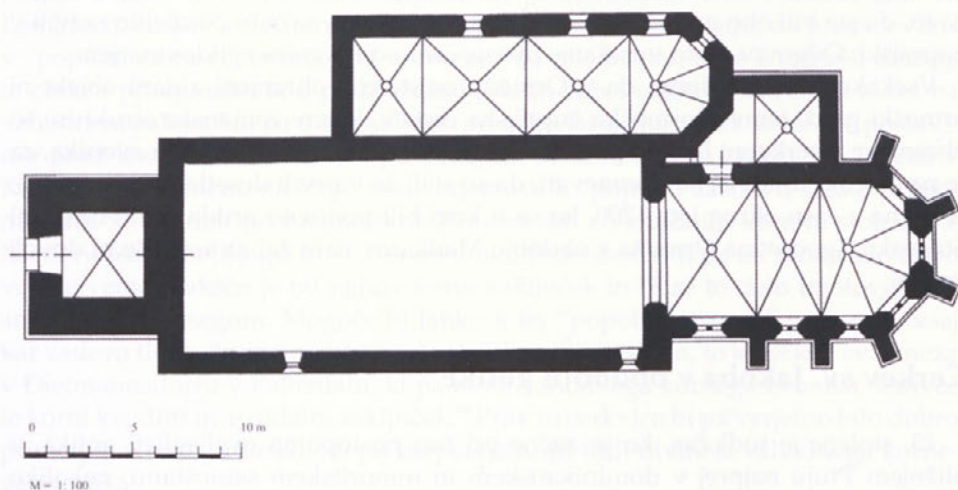
Slika 13: Ormož, župnijska cerkev sv. Jakoba st., 15. stoletje - tloris 3. Risal: B. Vnuk, september 2004
