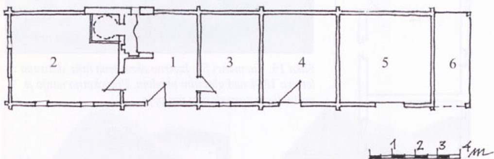
Skica 2: Lahonci 21: Tloris stegnjenega doma: 1. veža »priklet« in kuhinja, 2. hiša s krušno pečjo, 3. shramba, 4. hlev, 5. skedenj, 6. listnik.
