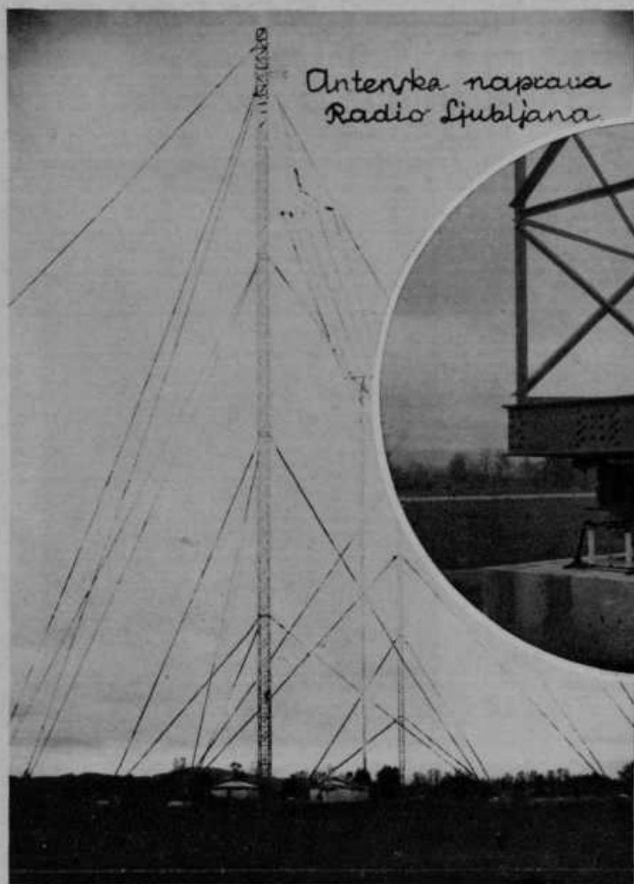
Oba antenska stolpa s peterožično anteno. Stolpa sta iz jekla ter visoka po 120 m.
