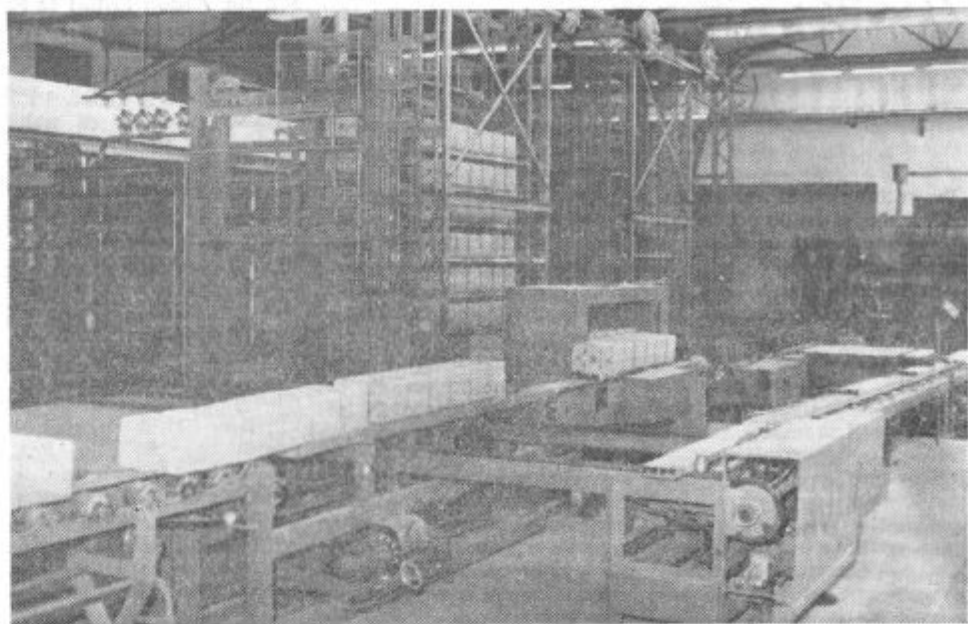
Novo naprave v obnovljeni tovarni EFE
