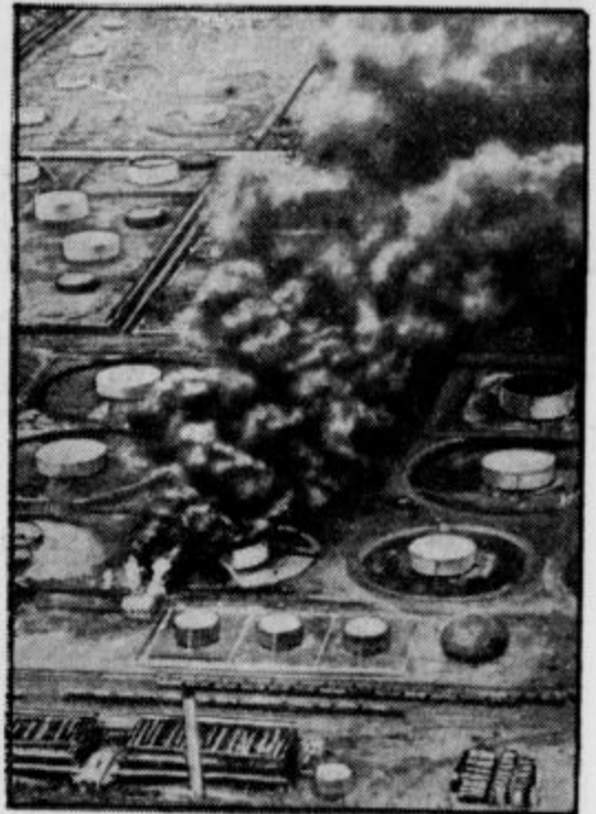
V petrolejski čistilnici v Whitingu je eksplodirala velika množina petroleja, da je bilo mahoma vse v ognju in črni oblaki dima. Več delavcev se je ponesrečilo. — Slika je posneta iz zrakoplova
